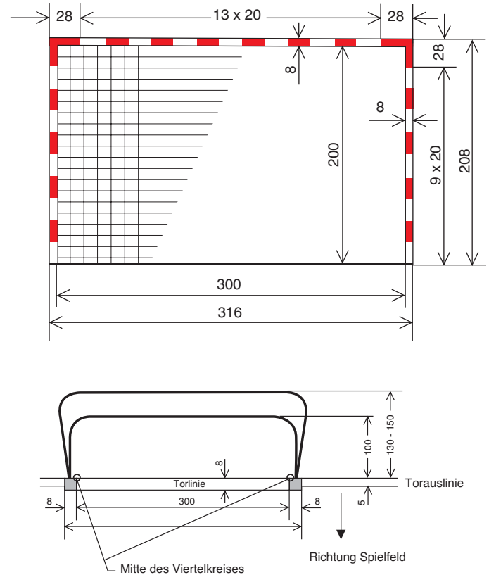
Abbildung 2a: Das Tor
